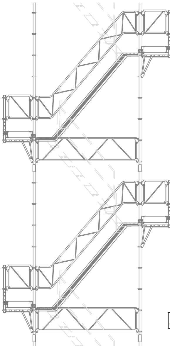
ELEVATION
