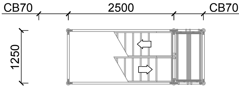
PLAN 'A'
